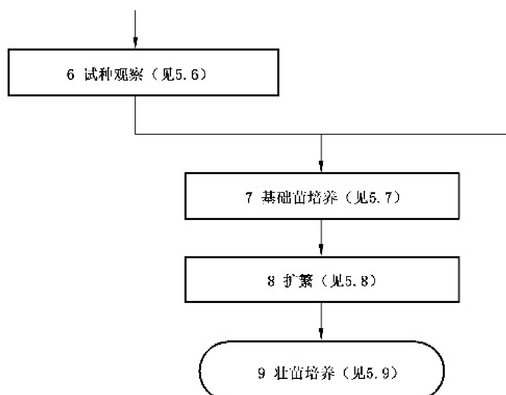
图1 马铃薯脱毒试管苗繁育程序流程图
